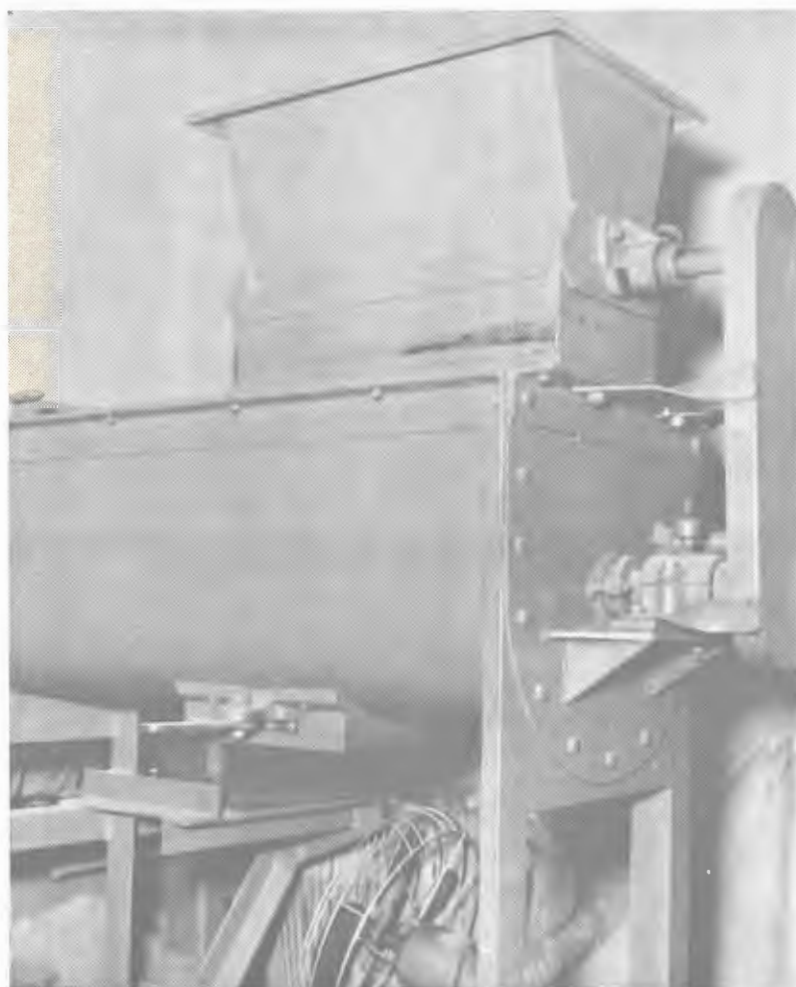
بوسیله این ماشین ، مواد سازنده هر قرص بمدت هشت روز مرتباً بهم زده شده و مخلوط میگردد .
